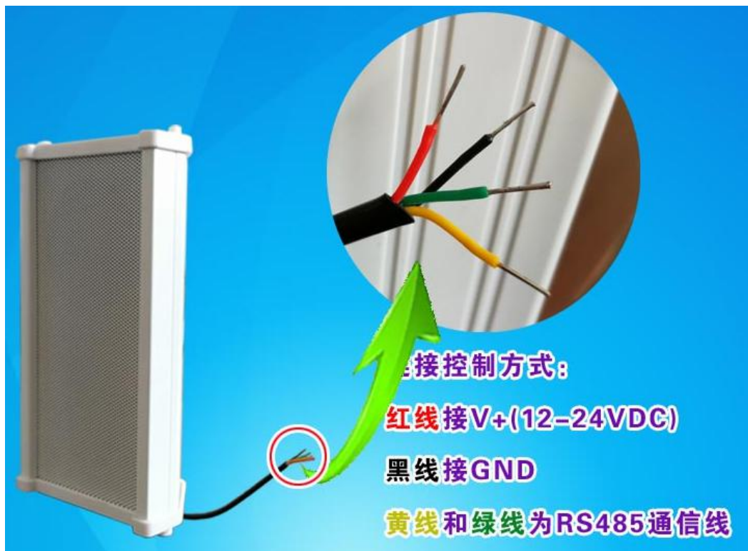
图 2 接线示意图
