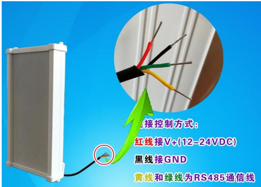
图 2 接线示意图
